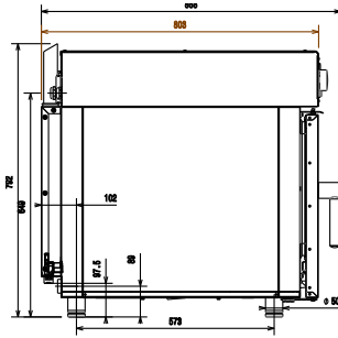
Oldalnézet
