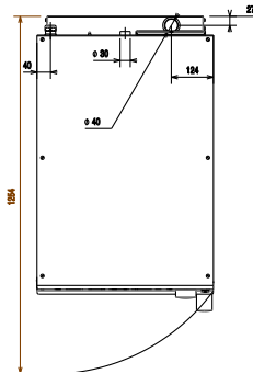
Felülnézet
